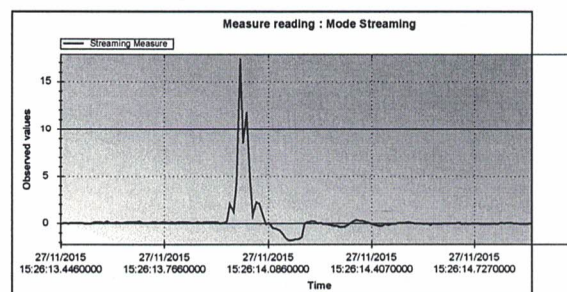
Figura 03 – Aceleração vertical
