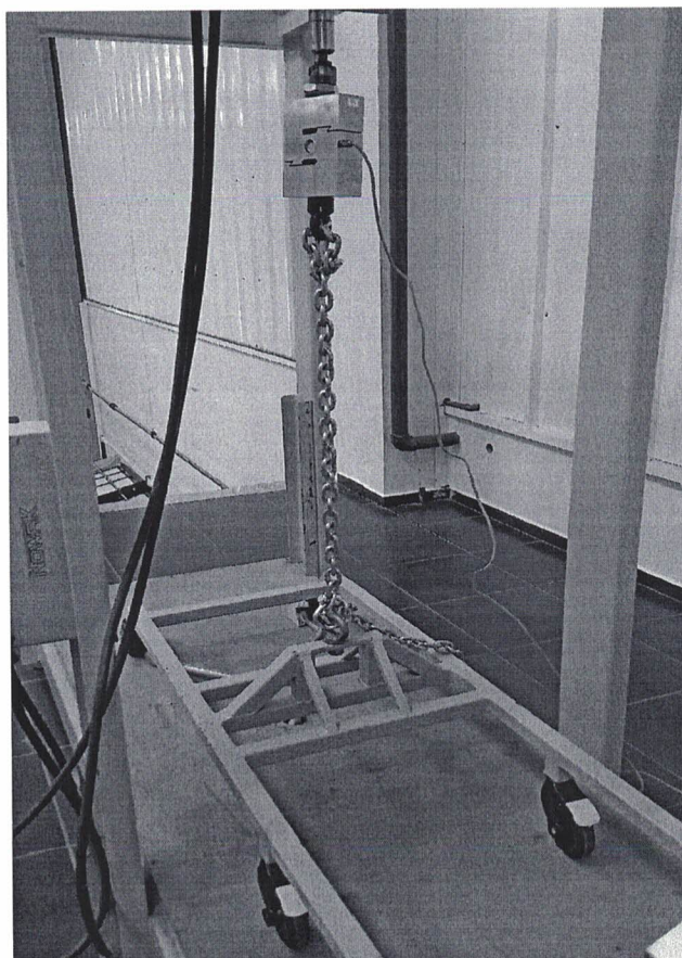
Foto 06 - Aplicação de carga no sentido vertical
