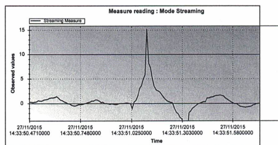
Figura 05 – Aceleração lateral
