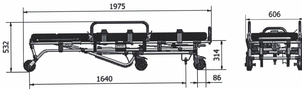
Figura 03 – Maca desarmada
