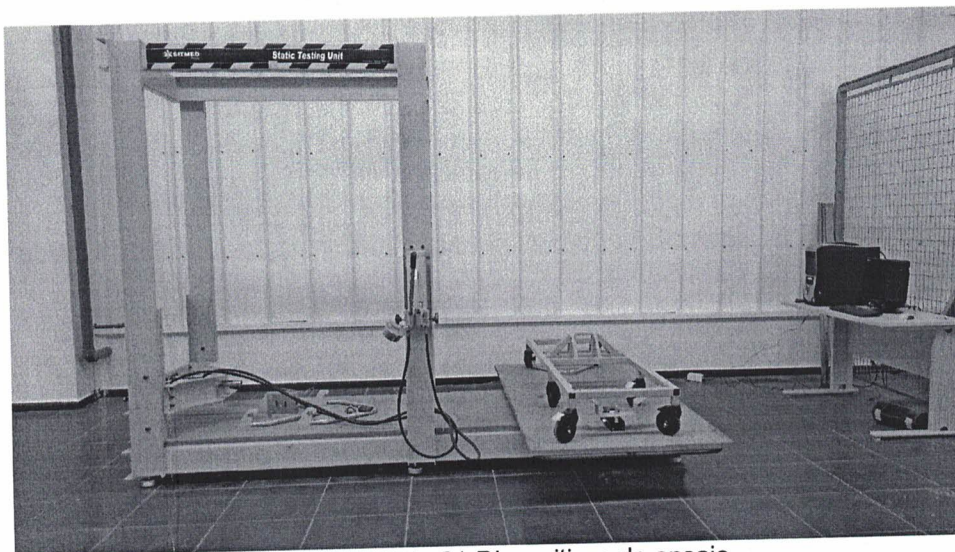
Foto 01-Dispositivos de ensaio
