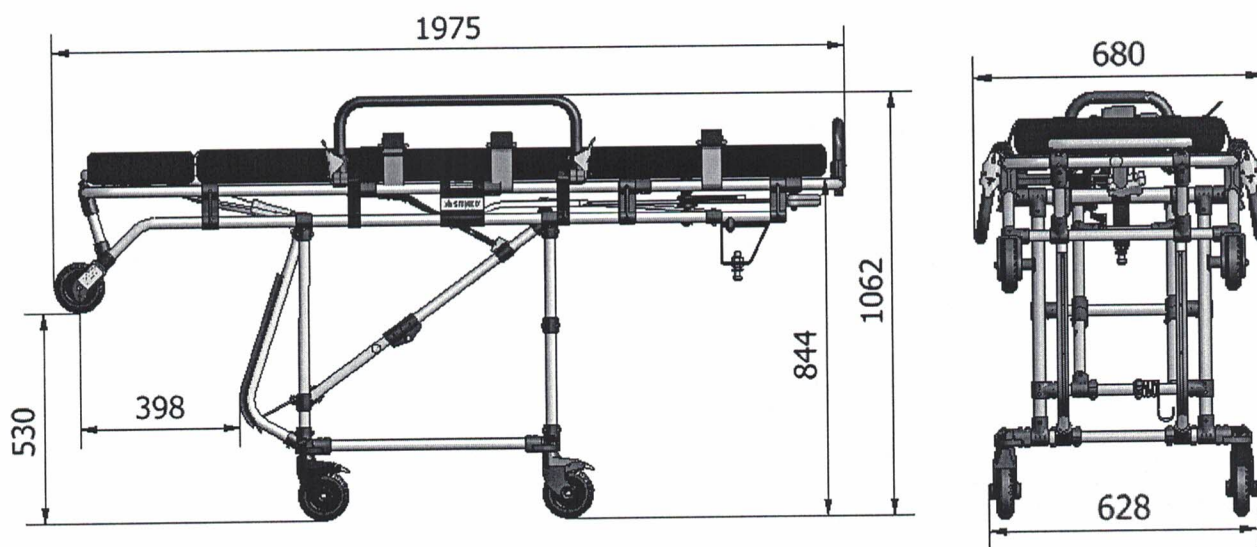
Figura 02 – Maca Armada
