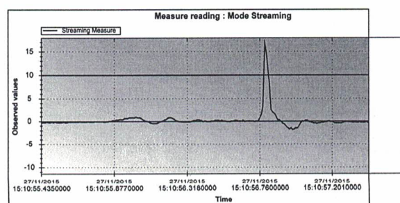
Figura 07 – Aceleração frontal
