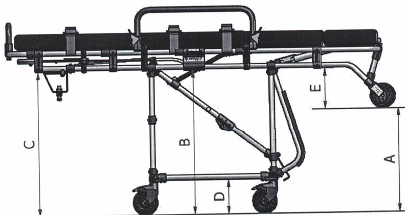
Figura 04 – Vista lateral
