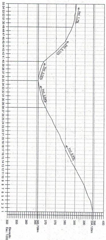
PERFIL LONGITUDINAL
