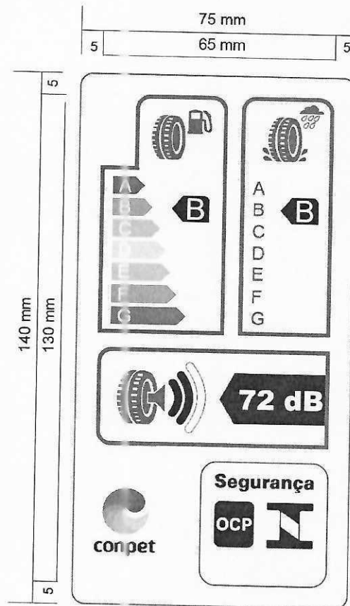
Figura 3- Formato e dimensões da ENCE para pneus novos, das Categorias C2, C3 e C4.
