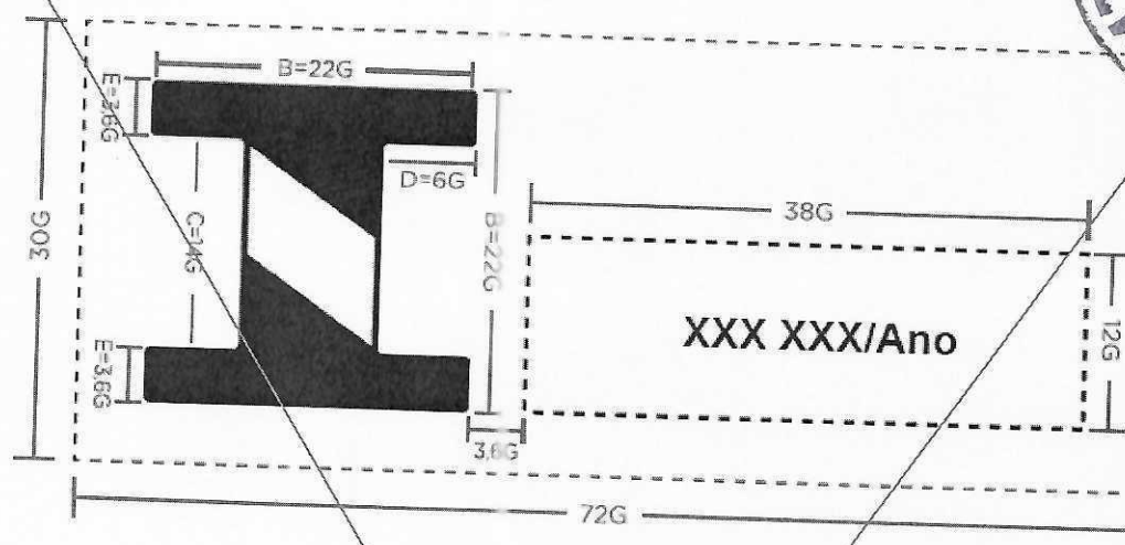
Figura 2 – Selo de Identificação da Conformidade para novas famílias de pneus
