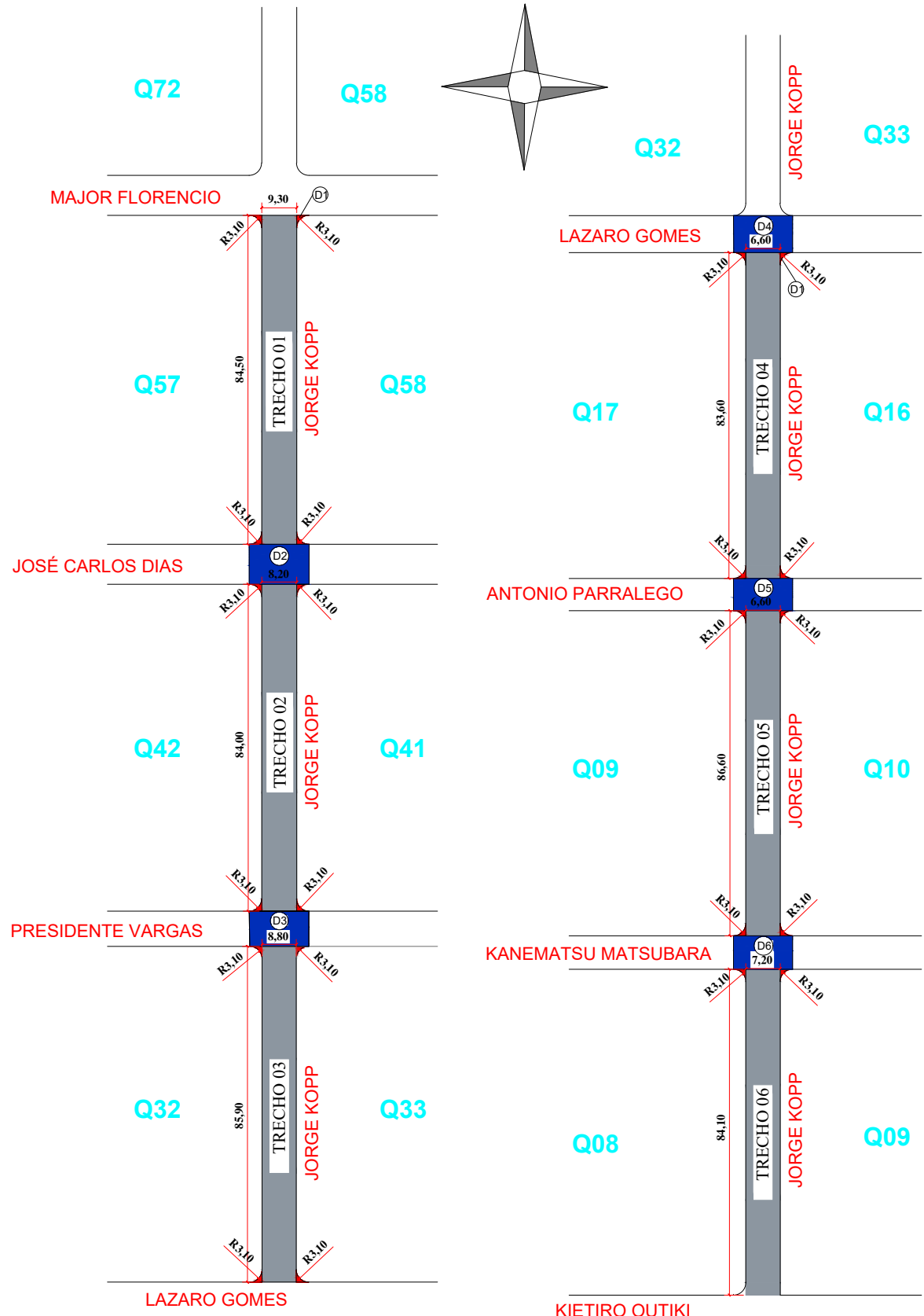
PLANTA DE INTERSEÇÕES Rua Jorge Kopp Trechos: 1, 2 e 3 ESC.: 1:2.000
