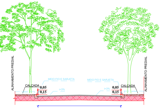
DETALHE CORTE TRANSVERSAL (Seção Transversal) SEM ESCALA
