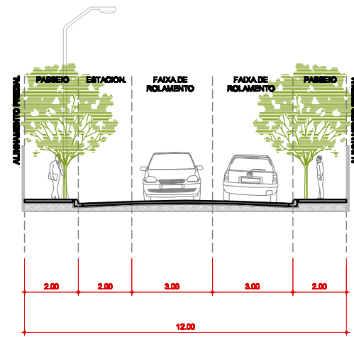
PERFIL VIA LOCAL
