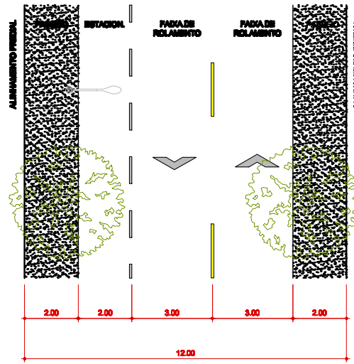
PLANTA VIA LOCAL
