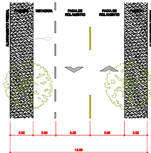
PLANTA VIA COLETORA
