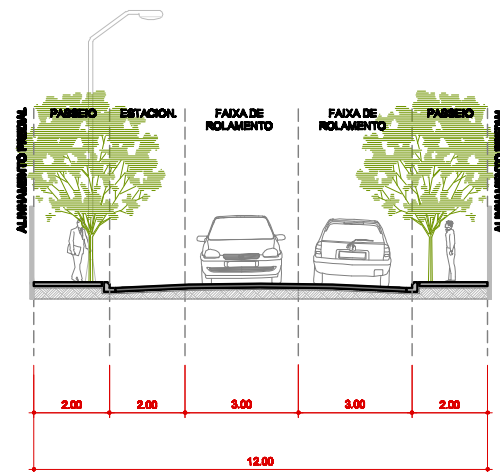
PERFIL VIA COLETORA
