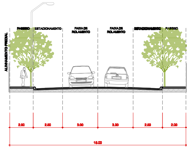
PERFIL VIA ESTRUTURAL
