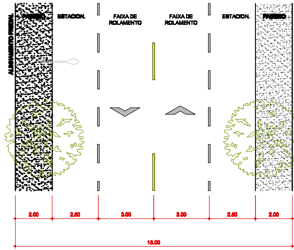
PLANTA VIA ESTRUTURAL
