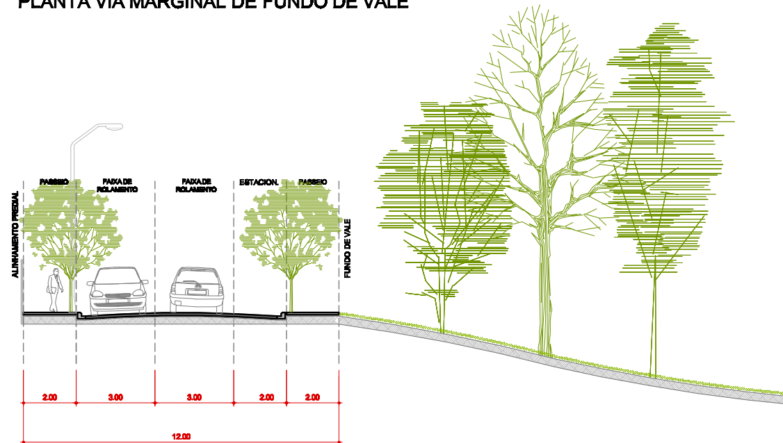
PERFIL VIA MARGINAL DE FUNDO DE VALE
