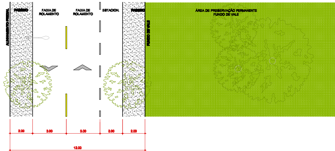
PLANTA VIA MARGINAL DE FUNDO DE VALE
