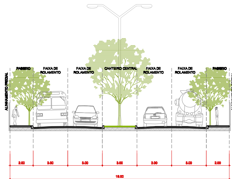
PERFIL VIA MARGINAL DE FUNDO DE VALE INDUSTRIAL
