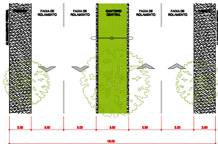
PLANTA VIA MARGINAL DE FUNDO DE VALE INDUSTRIAL
